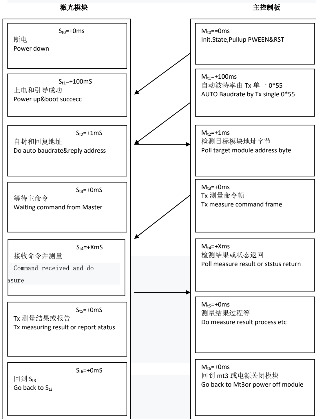
图 5-1 控制流
