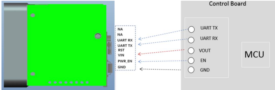
图 4-1 模块引脚
