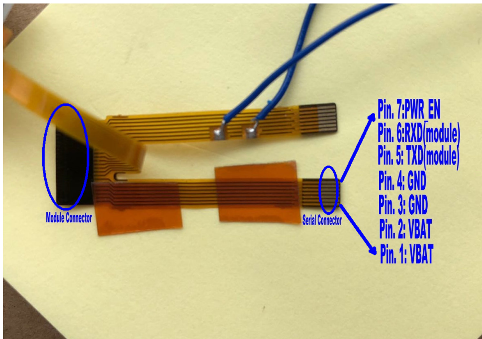
图 4-4 FPC 连接器
