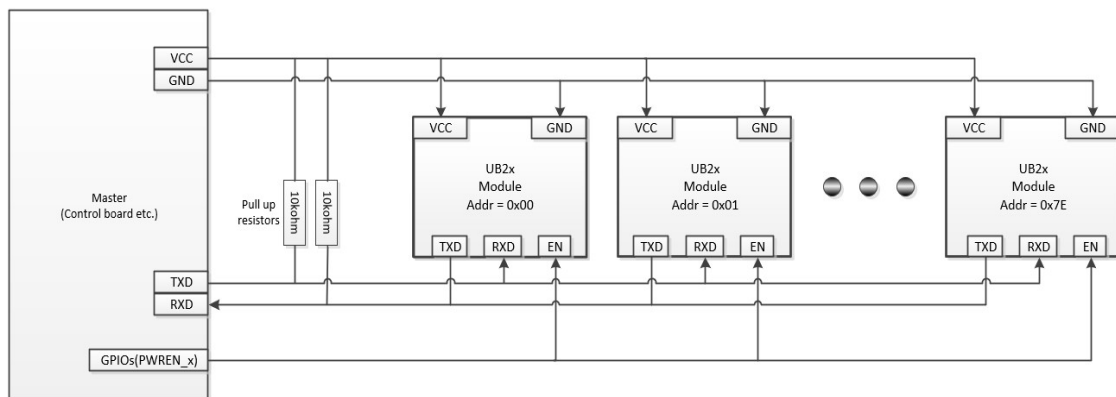
图 4-2 多模块接线
