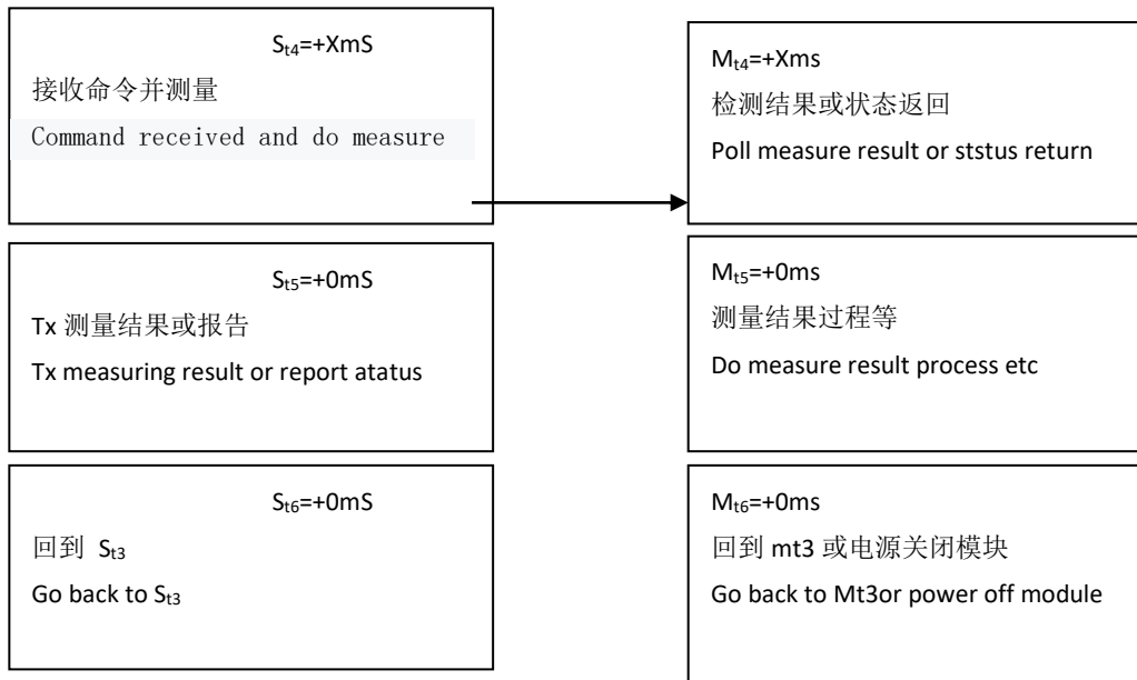
图 5-1 控制流程
